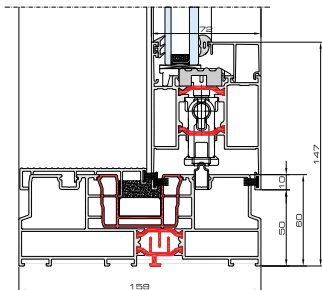
Kolos HI mit zwei Schienen vertikaler Querschnitt
