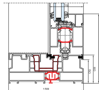
KOLOS HI mit zwei Schienen horizontaler Querschnitt
